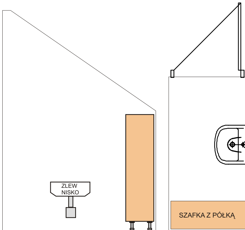
12/1. Szafka z półką wymiary: szer. 95 cm, wys. 145 cm, gł. 35 cm
